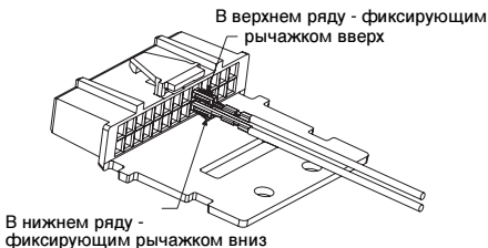
Рисунок 2. Ориентация наконечника
